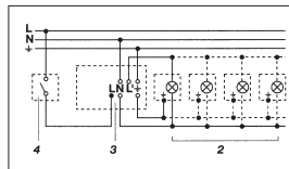
1. Svjetiljka bez postojećeg nulnog vodiča
