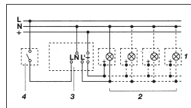
2. Светильник с имеющимся нулевым проводом
