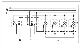
4. Pieslēgums ar maiņas slēdzi ilgstošā apgaismojuma un automātikas režīmam
