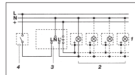
2. Svjetiljka s postojećim nulnim vodičem
