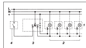
2. Svietidlo s nulovým vodičom
