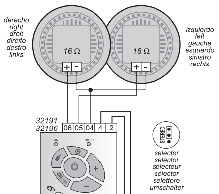
PUPITRE DE LLAMADAS INTERCOM MICROPHONE BASE PUPITRE D'APPELS MESA DE COMANDO DE CHAMADAS BASE DI CHIAMATE SPRECHSTELLE
